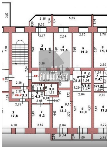
План 2 этажа
